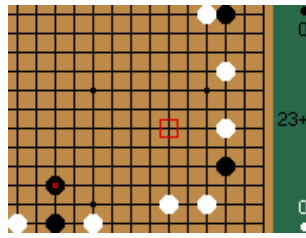
Figure 12.11.: Goban
